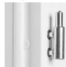
Zawias dwuczopowy Ilość sztuk: • 3 szt. dla wszystkich szerokości drzwi
