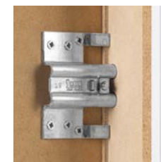
Stalowa kieszeń mocująca zawias. Zawiera ząbkowany zacisk eliminujący odkształcenie się zawiasów podczas użytkowania drzwi. Występuje tylko w ościeżnicy regulowanej.
